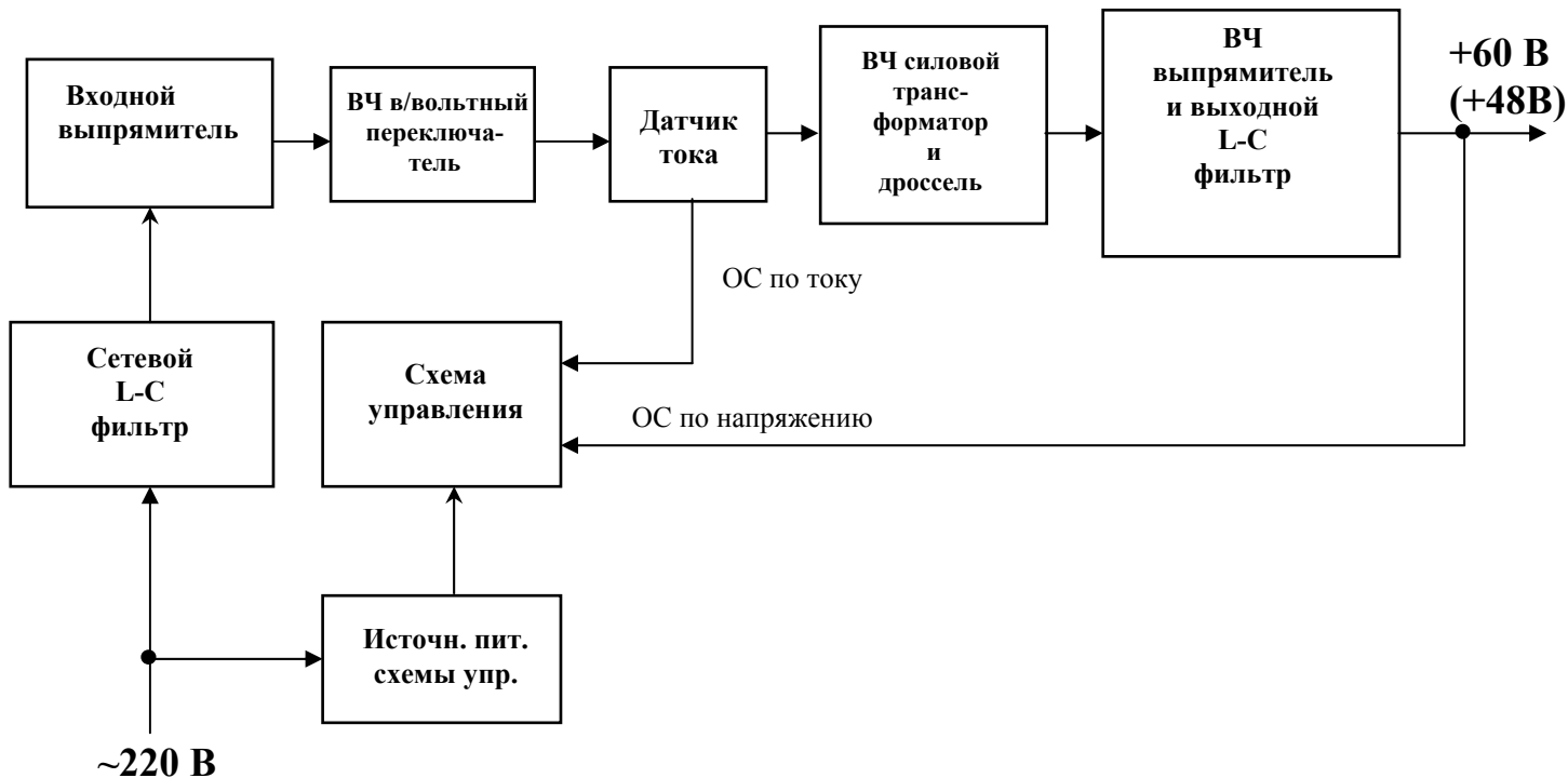
Рис.1. Структурная схема ИПС-950.
